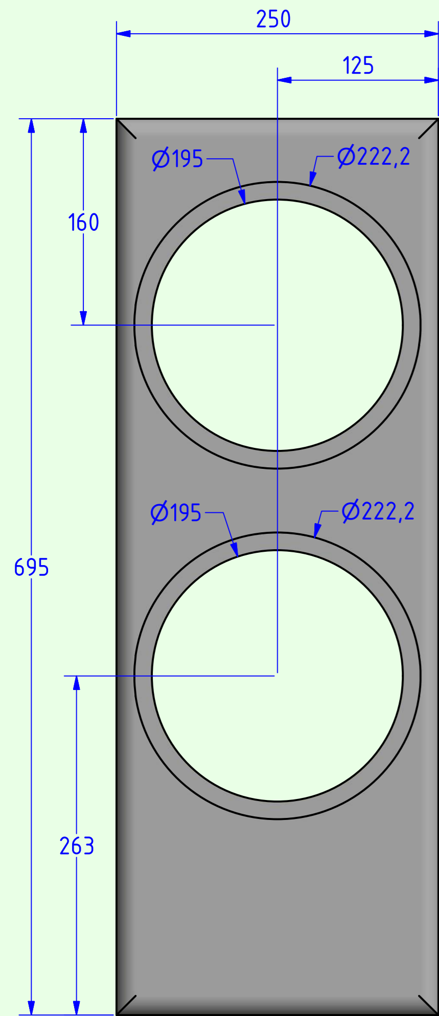
äußere Schallwand
