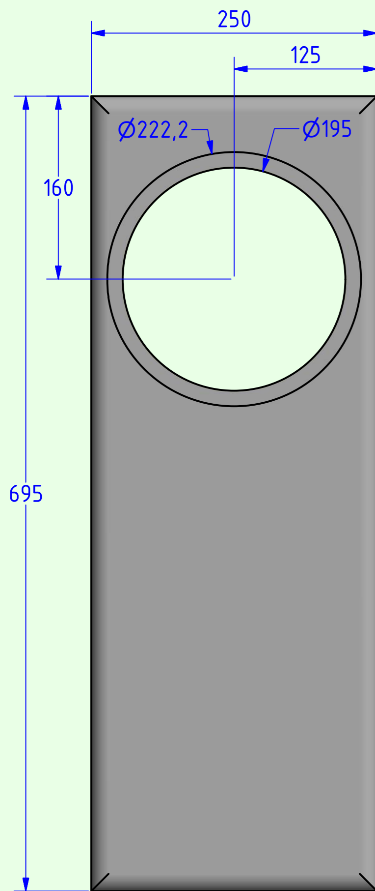
äußere Schallwand
